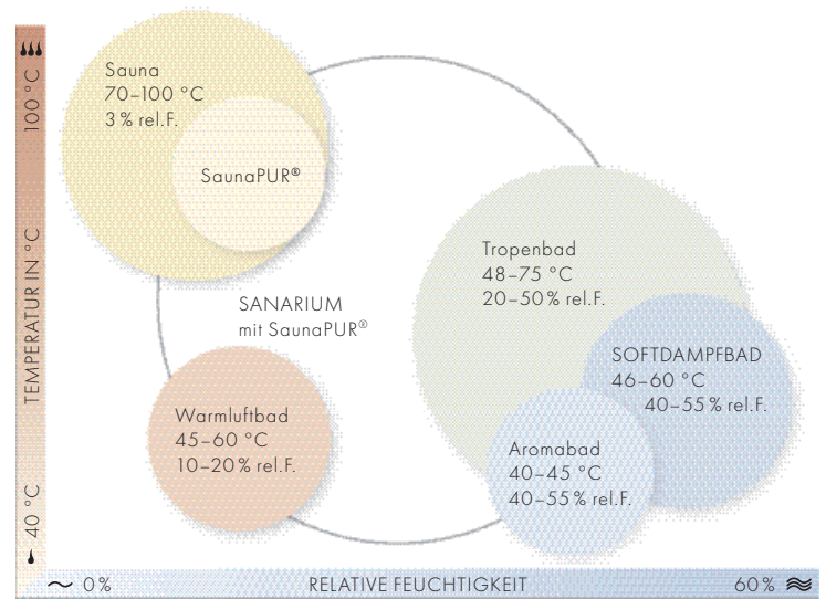
Das SANARIUM mit SaunaPUR® bietet fünf unterschiedliche Klimazonen.
