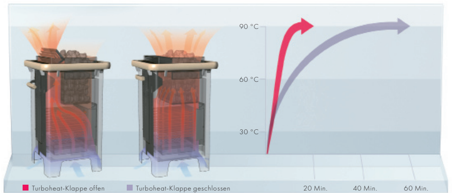
Dank Turboheat-Funktion sind 90 °C in der Sauna in nur 20 Minuten erreicht (Ausgangssituation: Raumtemperatur 20 °C).
